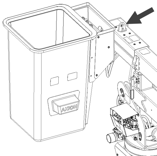
Ojal Arnés de Seguridad
