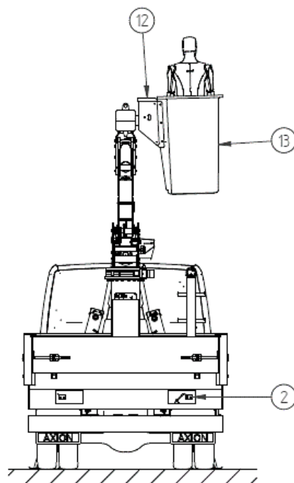
Vista Posterior Equipo BRX4313 doble aislado + Vehículo – Identificación de Partes
