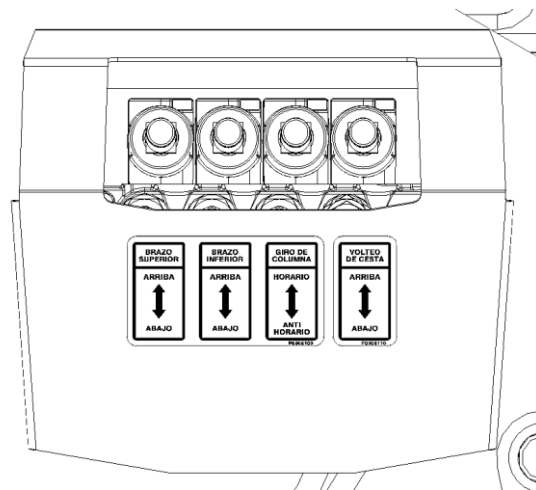
Controles de Columna
