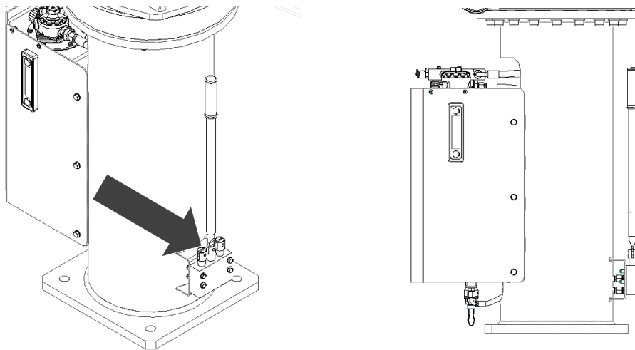
Bomba manual de emergencia
