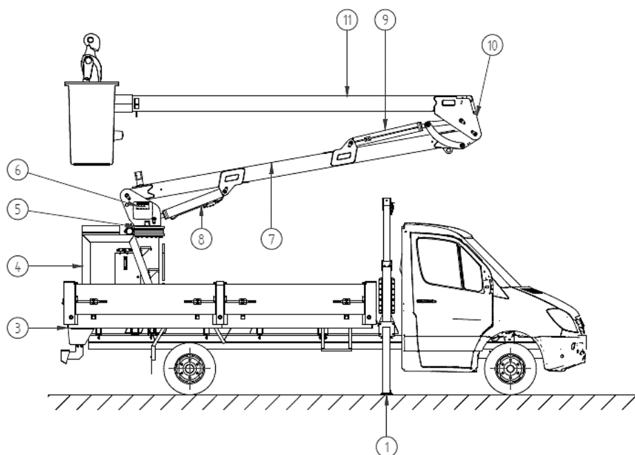
Vista Lateral Equipo BRX4313 doble aislado + Vehículo – Identificación de Partes
