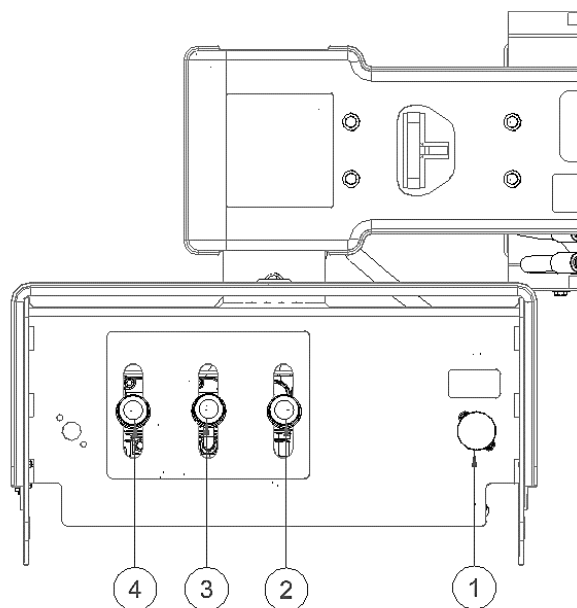
Controles de Barquilla
