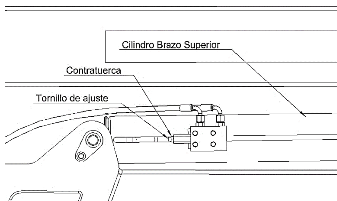
Válvula Honding Brazo Superior
