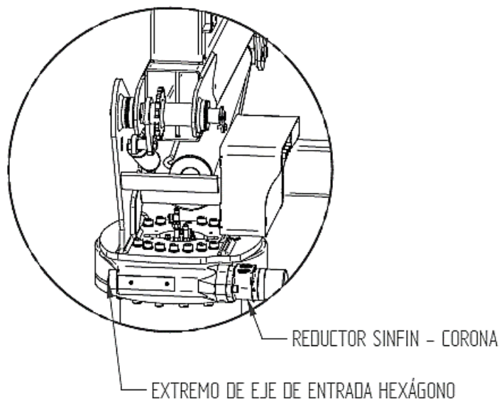
Rotación de Columna
